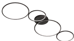
Deckenleuchte · Ceiling lamp ↔ 97 x 34,3 cm, ↑ 5,5 cm incl. SMD-LED, 37 W 4.800 lm, 3.000 K
