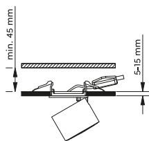
Strahler · Spot Ø 8,7 cm, ↓ 12 cm excl. 1 x GU10, max. 35 W
