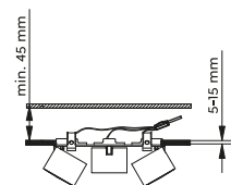
Strahler · Spot ↔ 27,3 x 8,7 cm, ↓ 12 cm excl. 3 x GU10, max. 35 W
