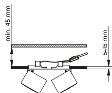
Strahler · Spot ↔ 18 x 8,7 cm, ↓ 12 cm excl. 2 x GU10, max. 35 W
